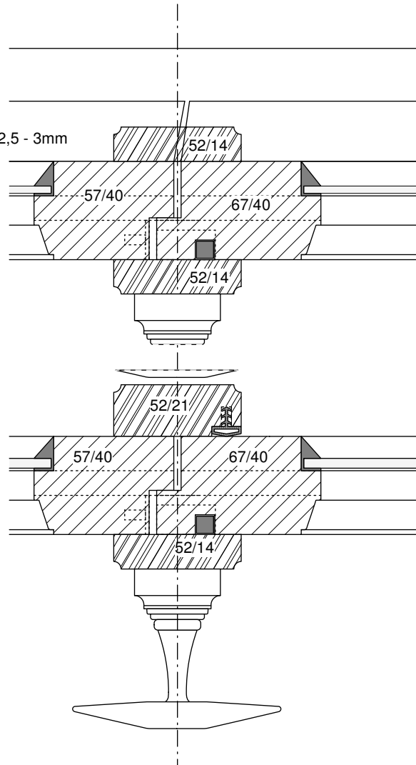
Salfeld / 1283 / KAF / M1:1 Höhenschnitt Stulpflügel
